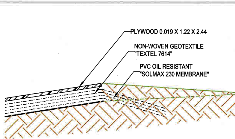
SECTION D-D D SCALE 1:15 F 2
