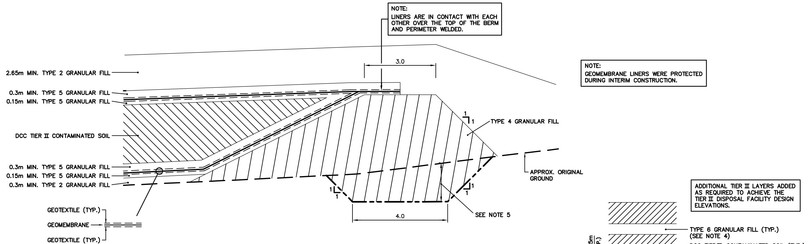
DETAIL 1 — N.T.S.
