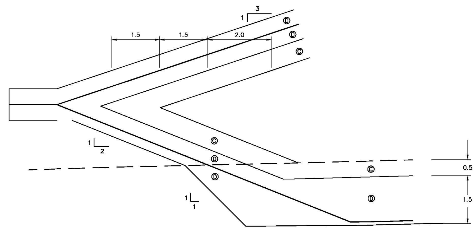
DETAIL N.T.S.
