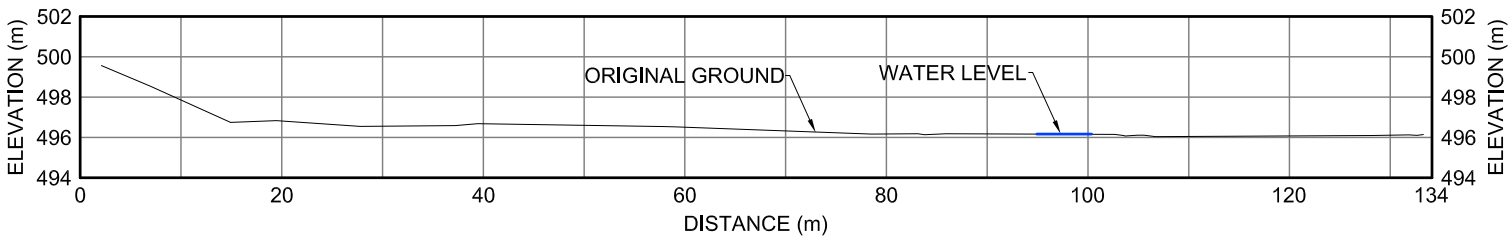
DS XII-23 CROSS-SECTION
