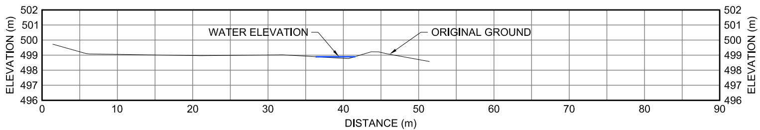
50DS XII-4 CROSS-SECTION
