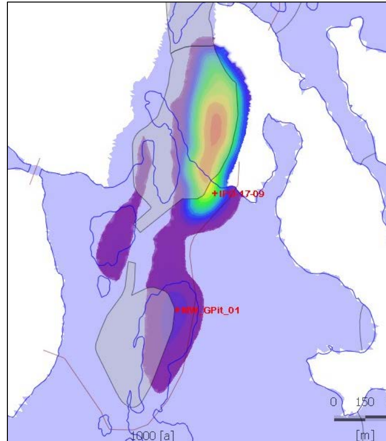
Slice 38 (-200 masl)
