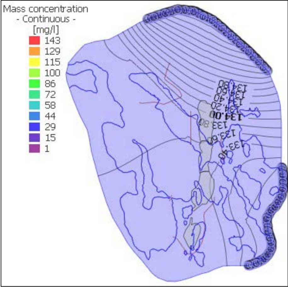
Slice 44 (-500 masl)
