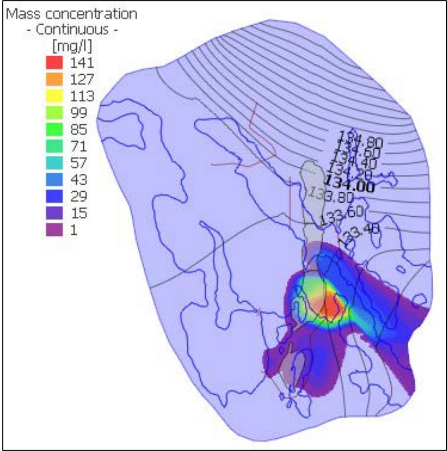
Slice 44 (-500 masl)
