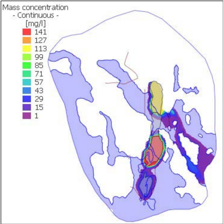
Slice 6 (120 masl)
