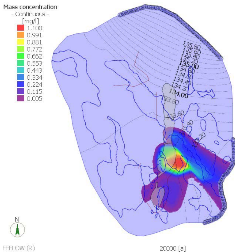
Slice 44 (-500 masl)
