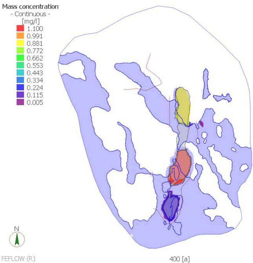
Slice 6 (120 masl)
