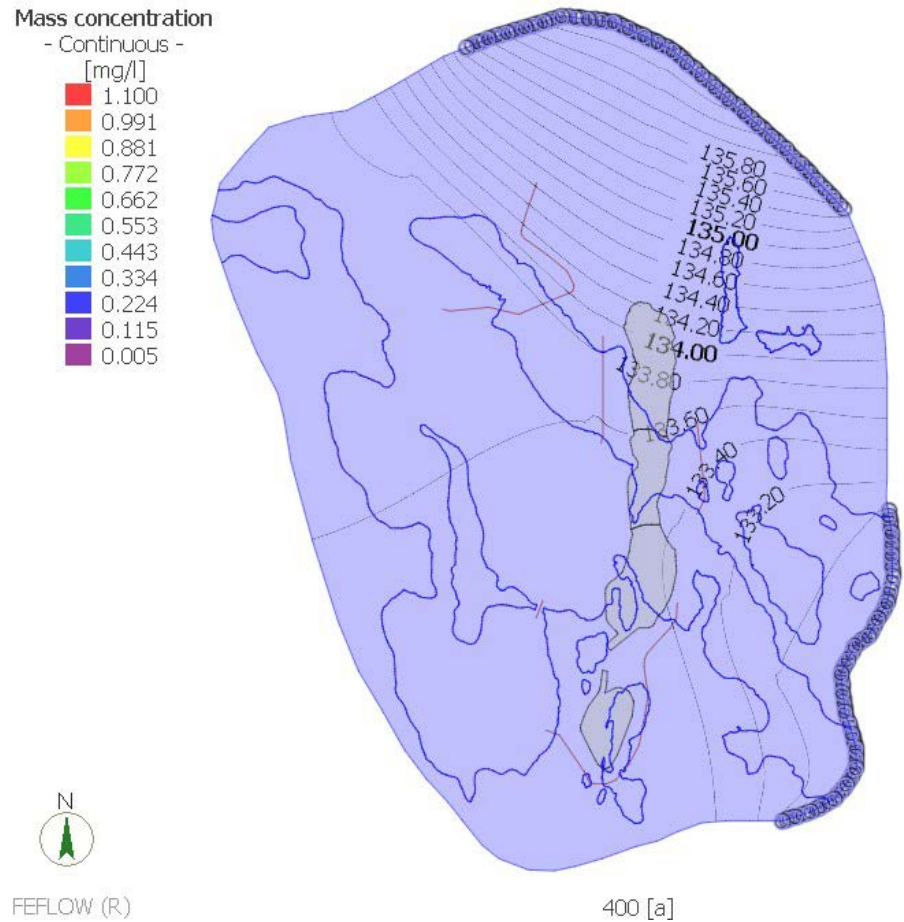
Slice 44 (-500 masl)
