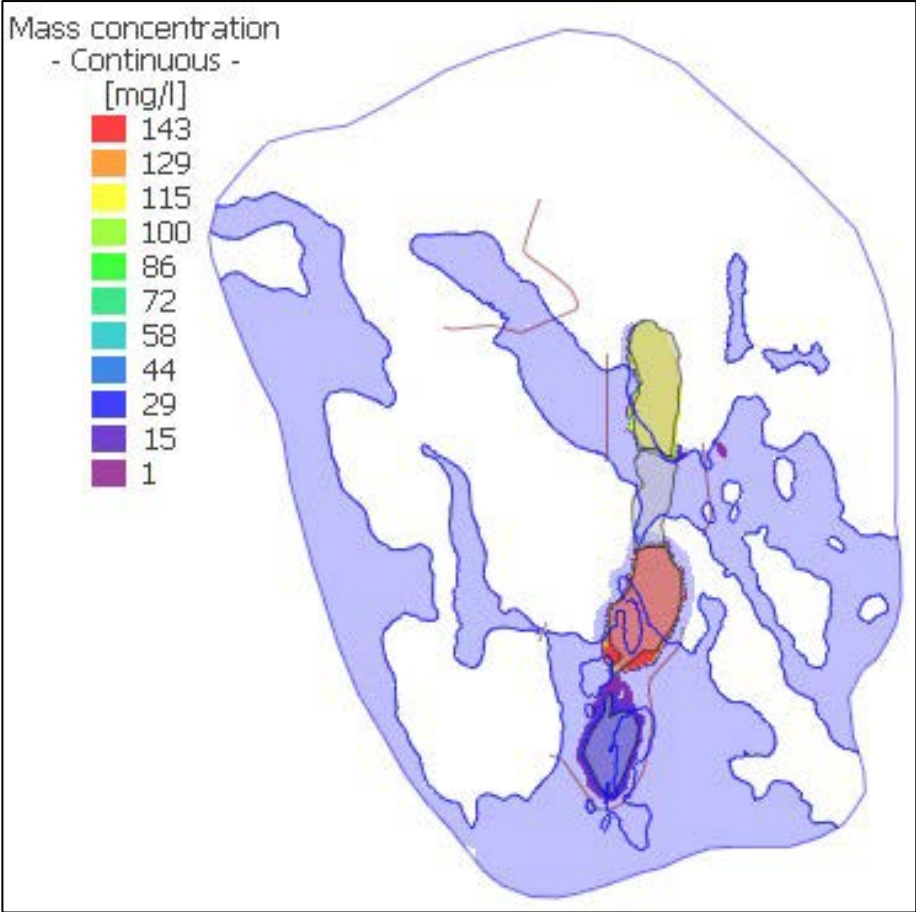
Slice 6 (120 masl)
