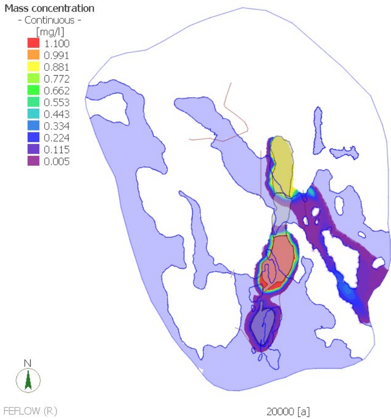
Slice 6 (120 masl)
