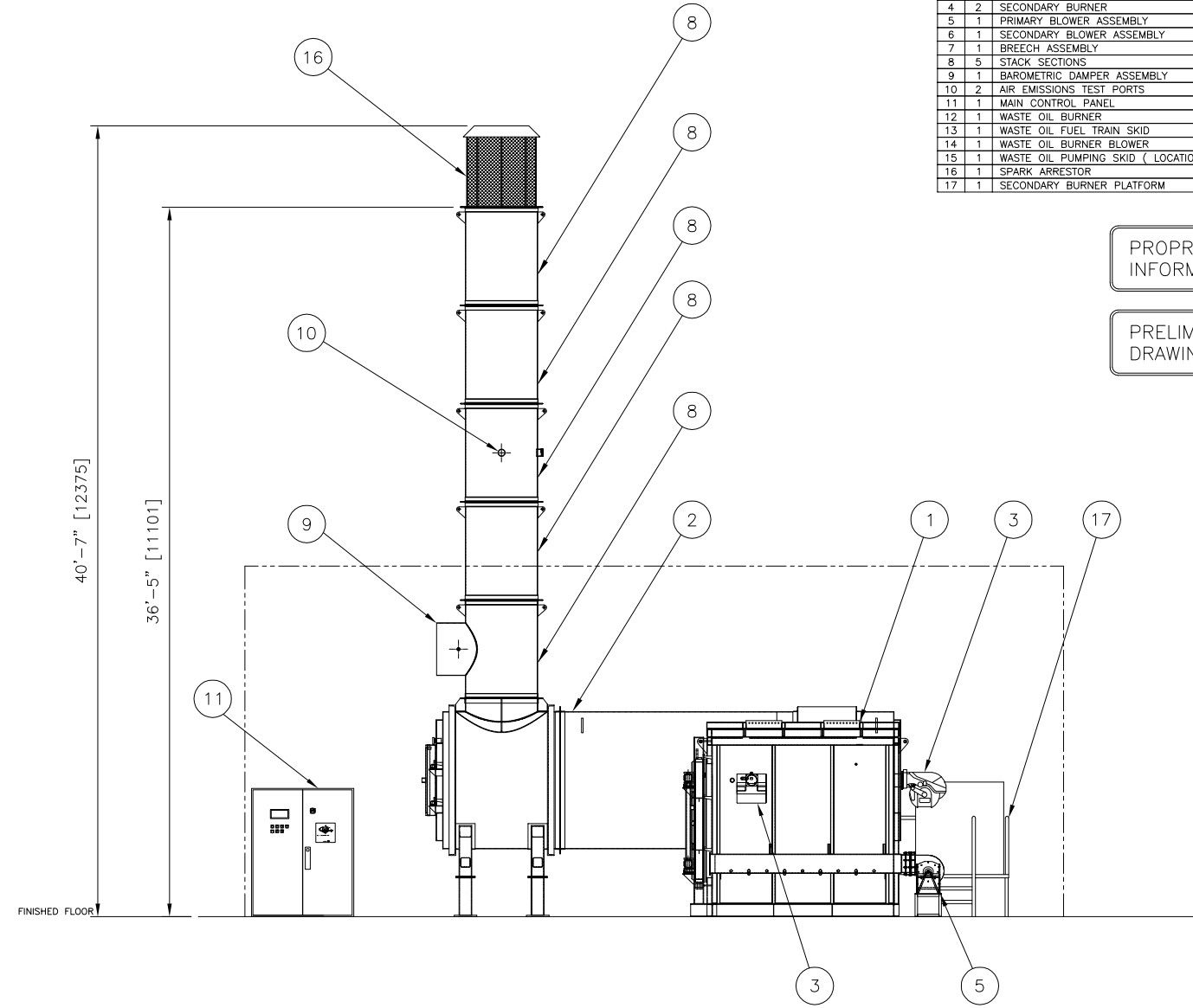
RIGHT ELEVATION
