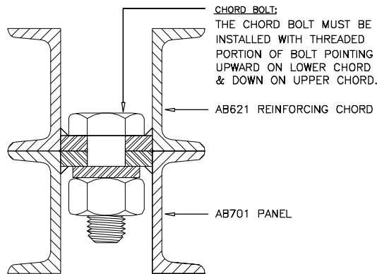
CHORD BOLT DETAIL SCALE: N.T.S.
