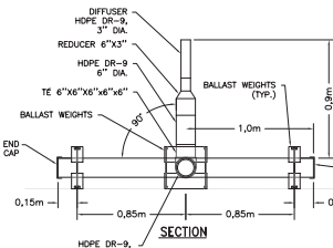
DETAILS - DIFFUSER Scale: 1:20
