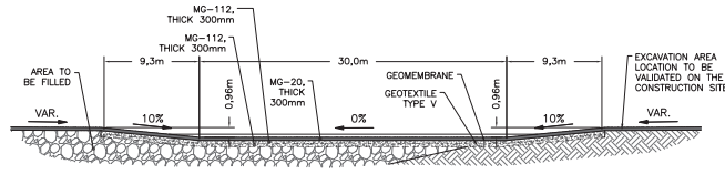
SECTION "B" - PAD Scale: 1:20
