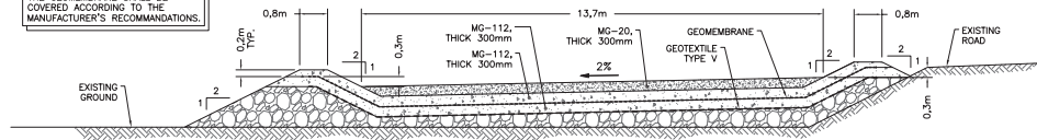
SECTION "A" - PAD Scale: NONE
