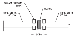
DETAIL - FLANGE Scale: 1:20
