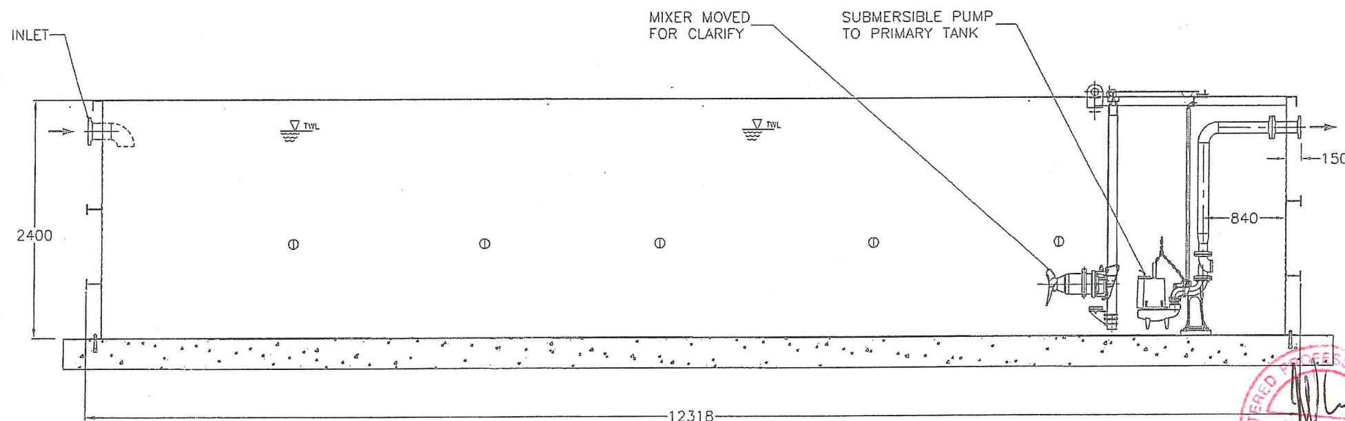
SECTION D-D
