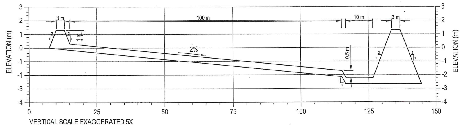
SECTION A-A
