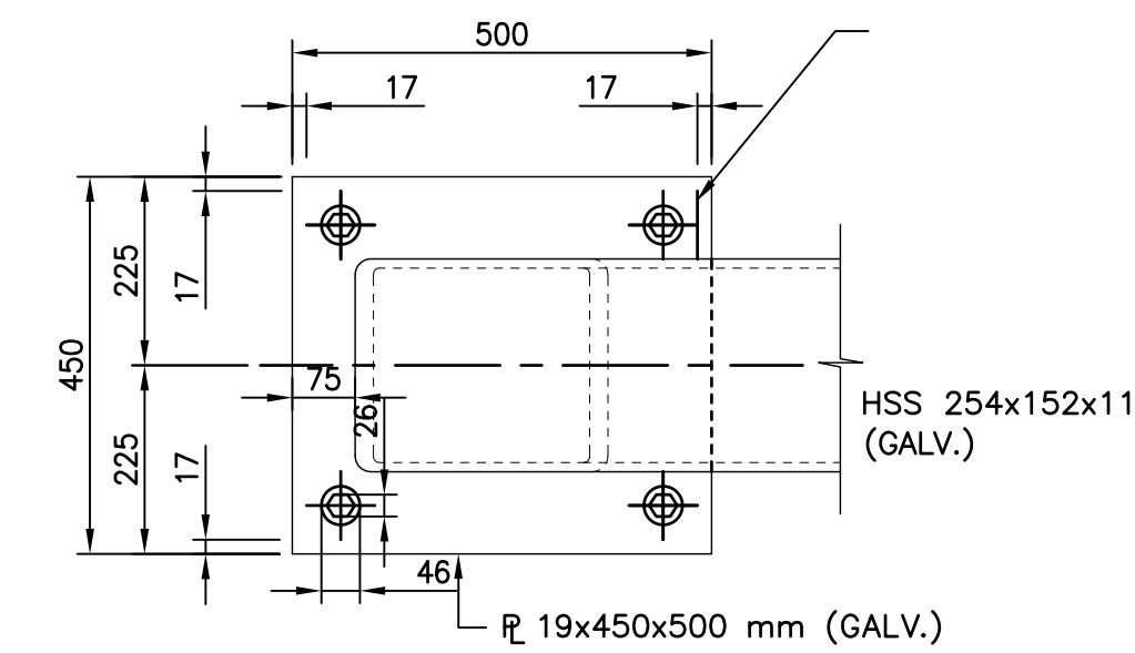
ANCHOR PLATE A SCALE: 1:10
