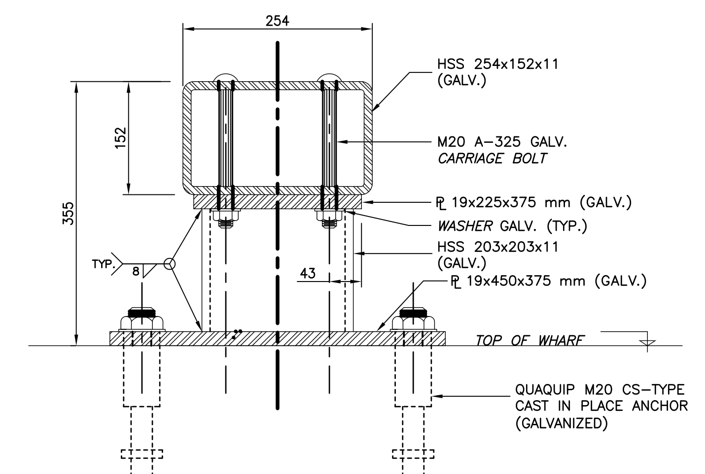
SECTION SCALE: 1:5
