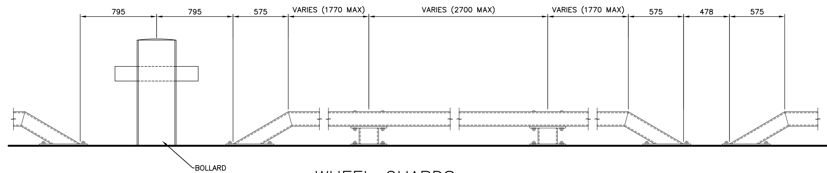
WHEEL GUARDS SCALE: 1:20
