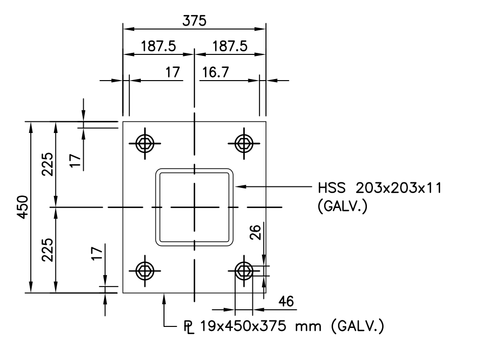
ANCHOR PLATE B SCALE: 1:10
