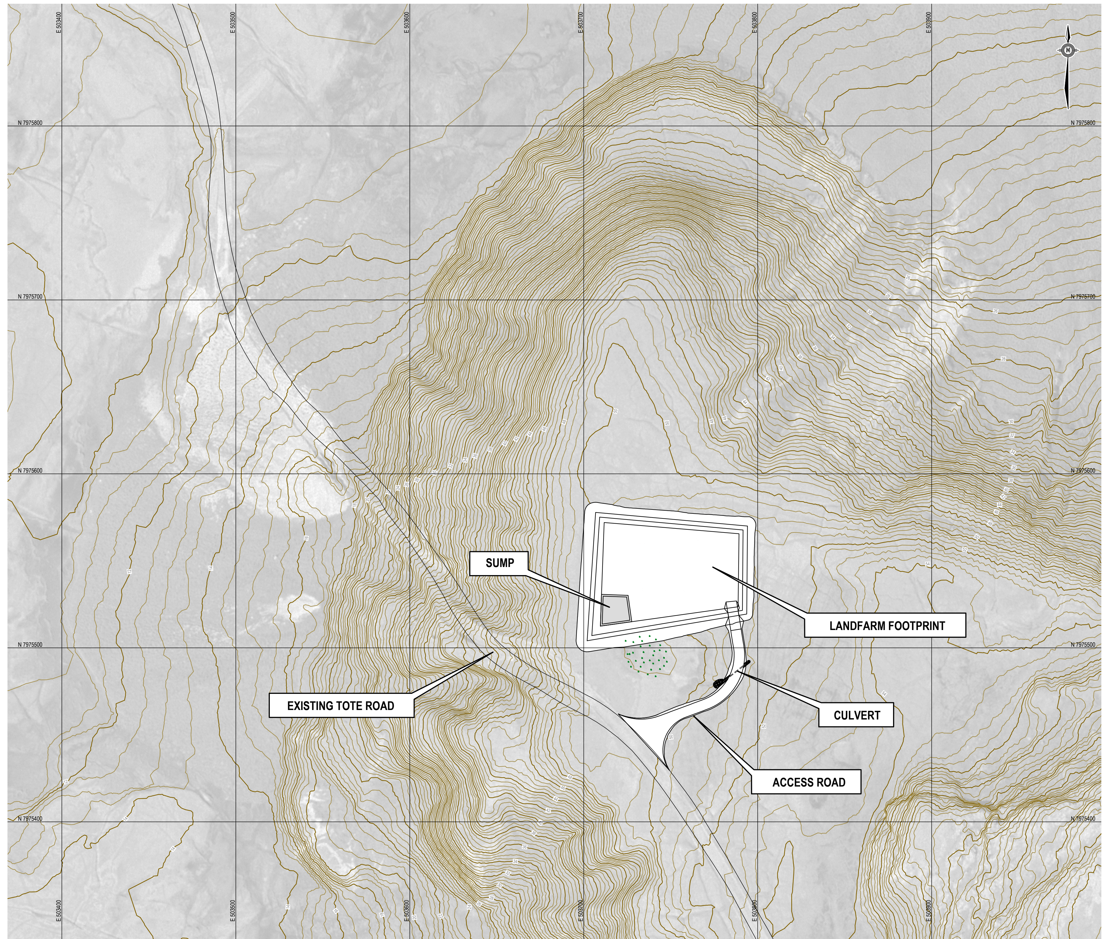
SCALE: 1: 1,250
