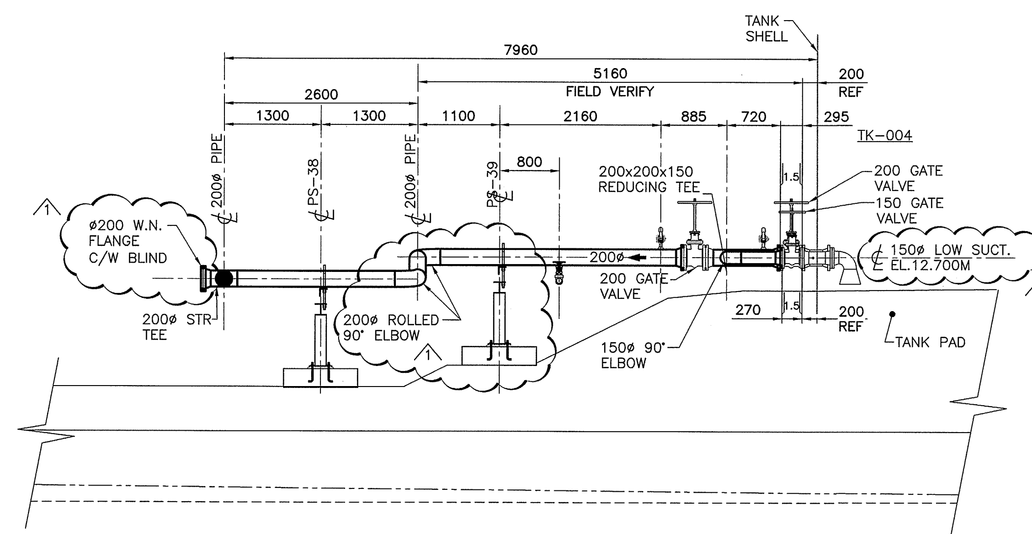
SECTION A 2613-60-012-000
