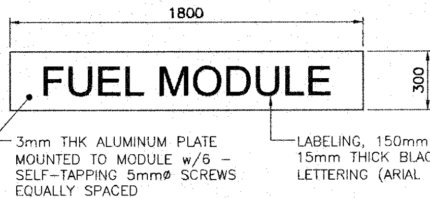
DETAIL FUEL MODULE SIGN SCALE: 1:20
