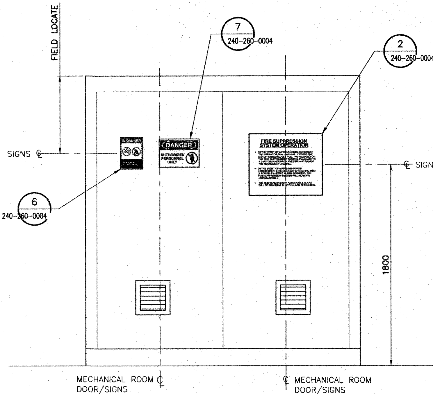
SECTION B-B DOOR SIGNAGE SCALE: 1:20
