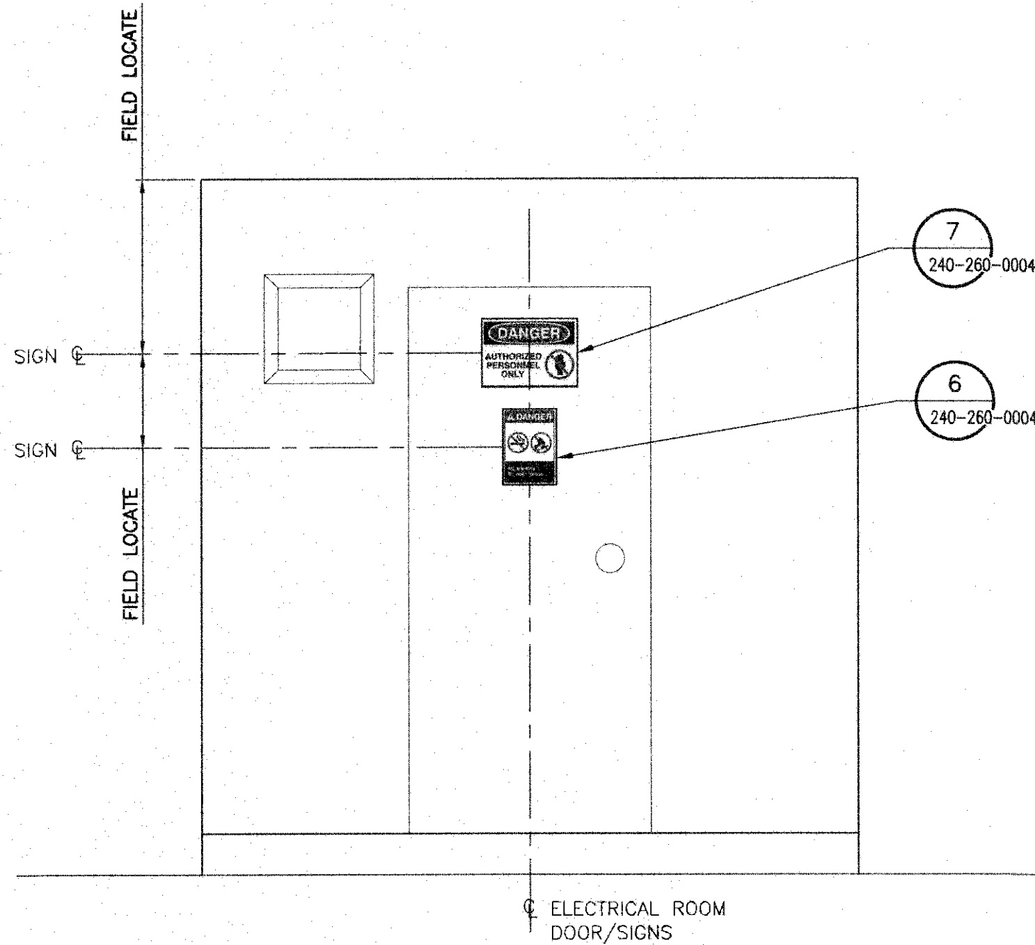
SECTION C-C DOOR SIGNAGE SCALE: 1:20
