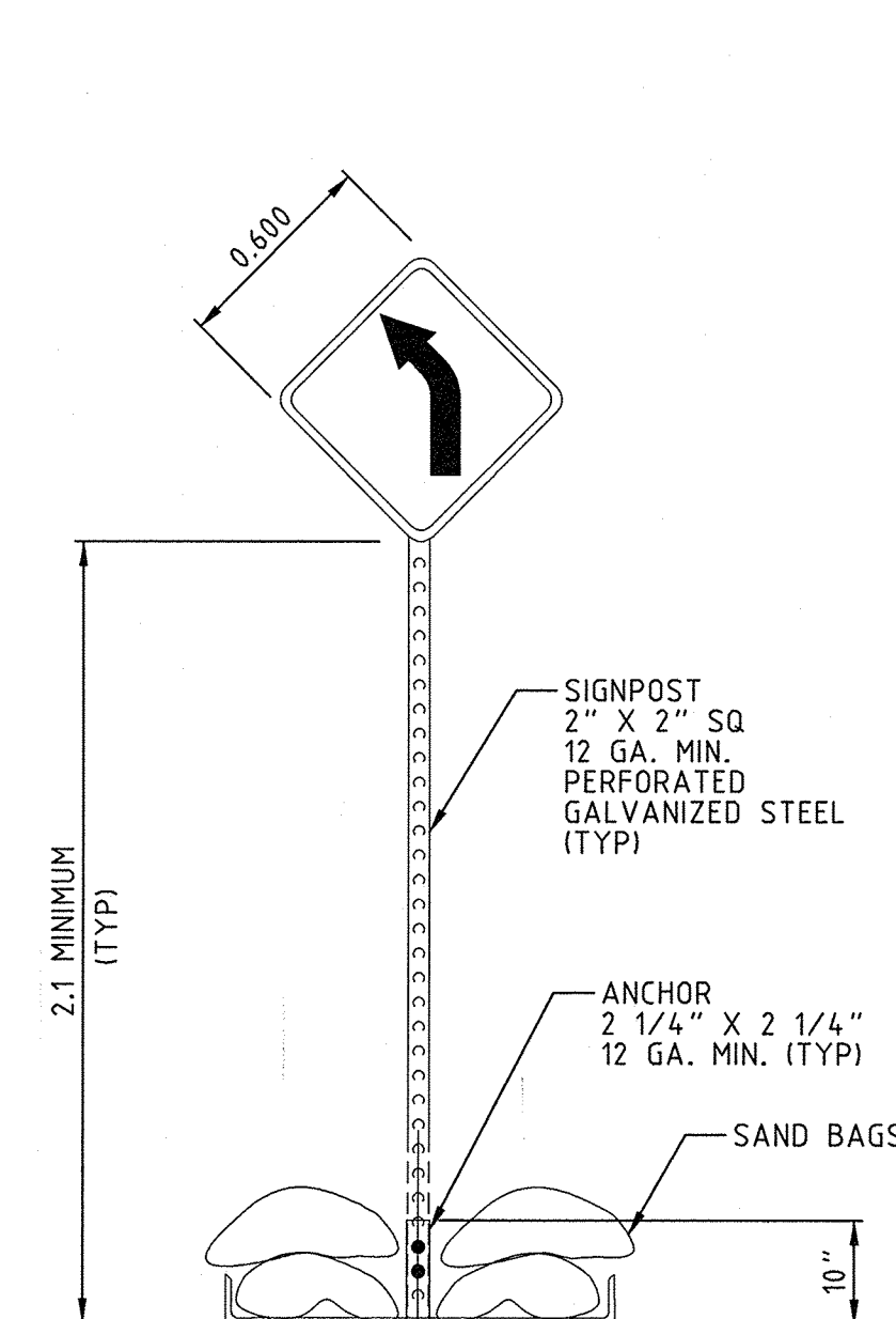
STEEL SIGN SINGLE BASE N.T.S.
