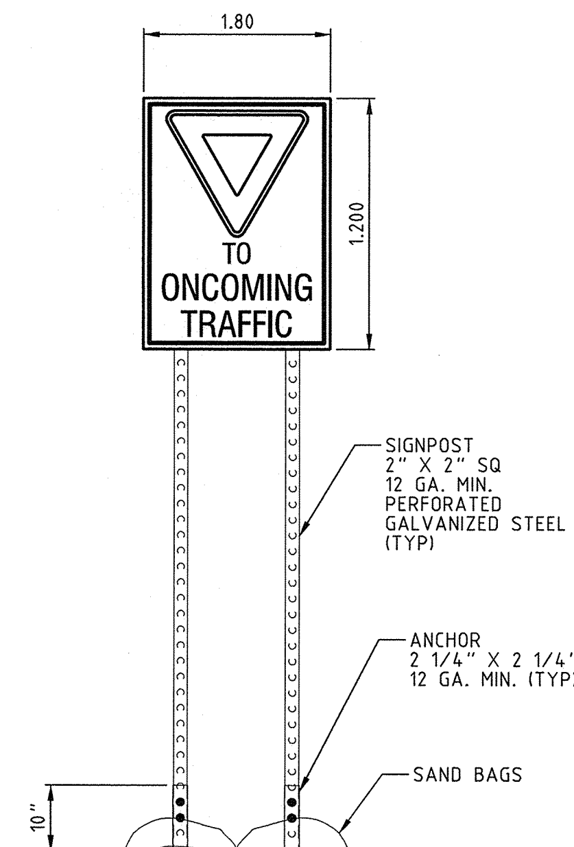
STEEL SIGN DOUBLE BASE N.T.S.
