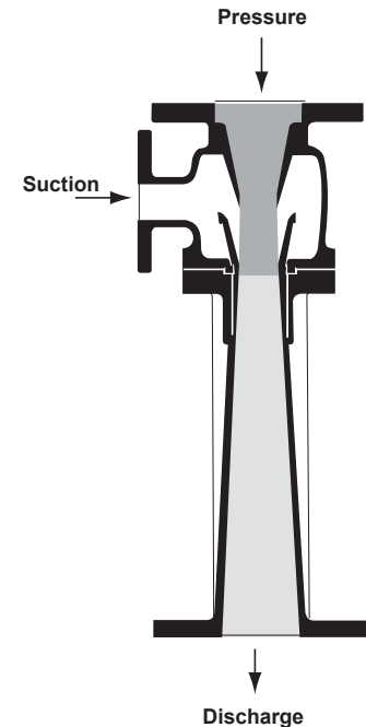
Fig. 11. FIG. 242 EDUCTOR.
