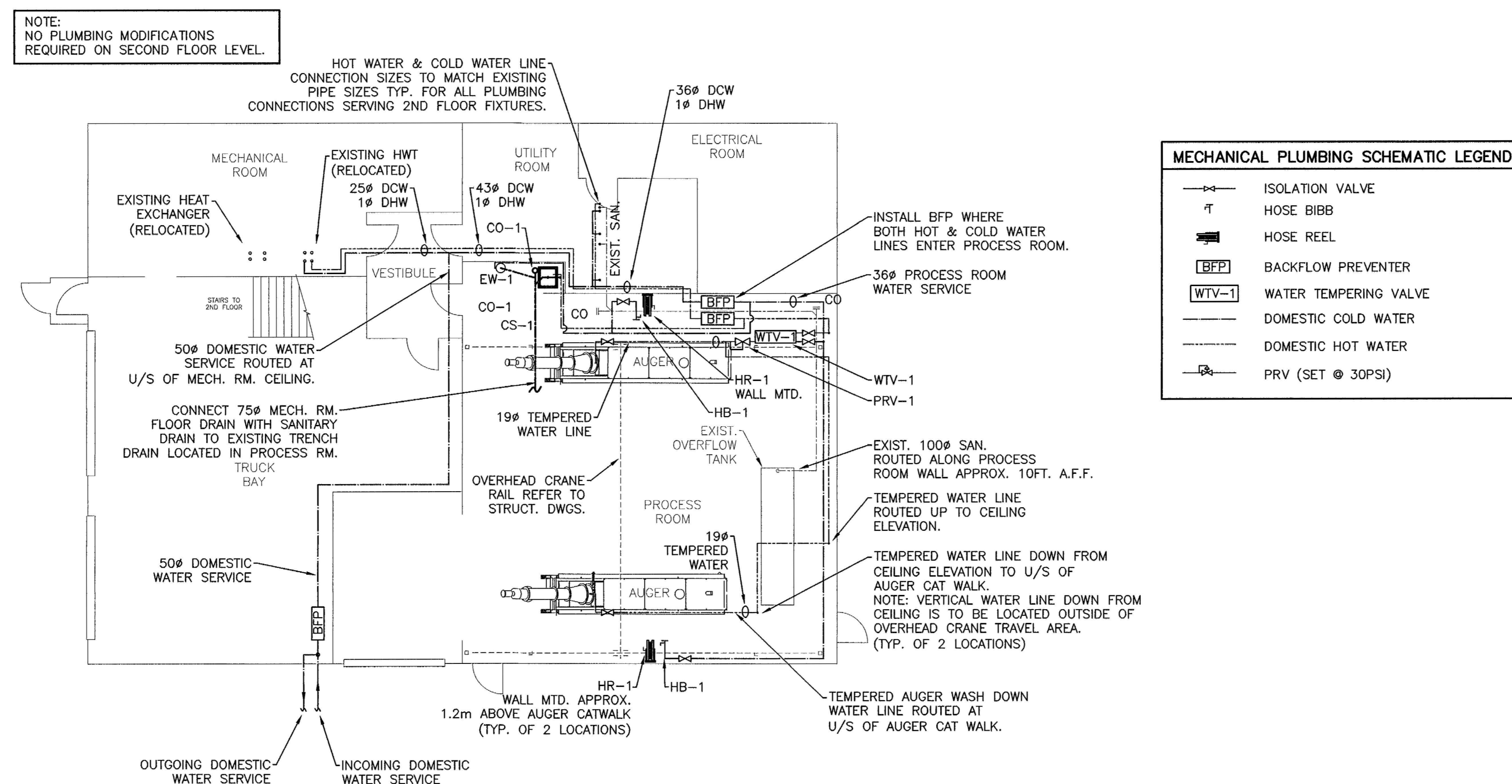
PLUMBING SCHEMATIC N.T.S.
