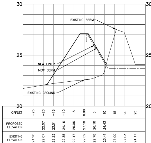
SECTION C (DWG NO. IGL-4 AND IGL-5)
