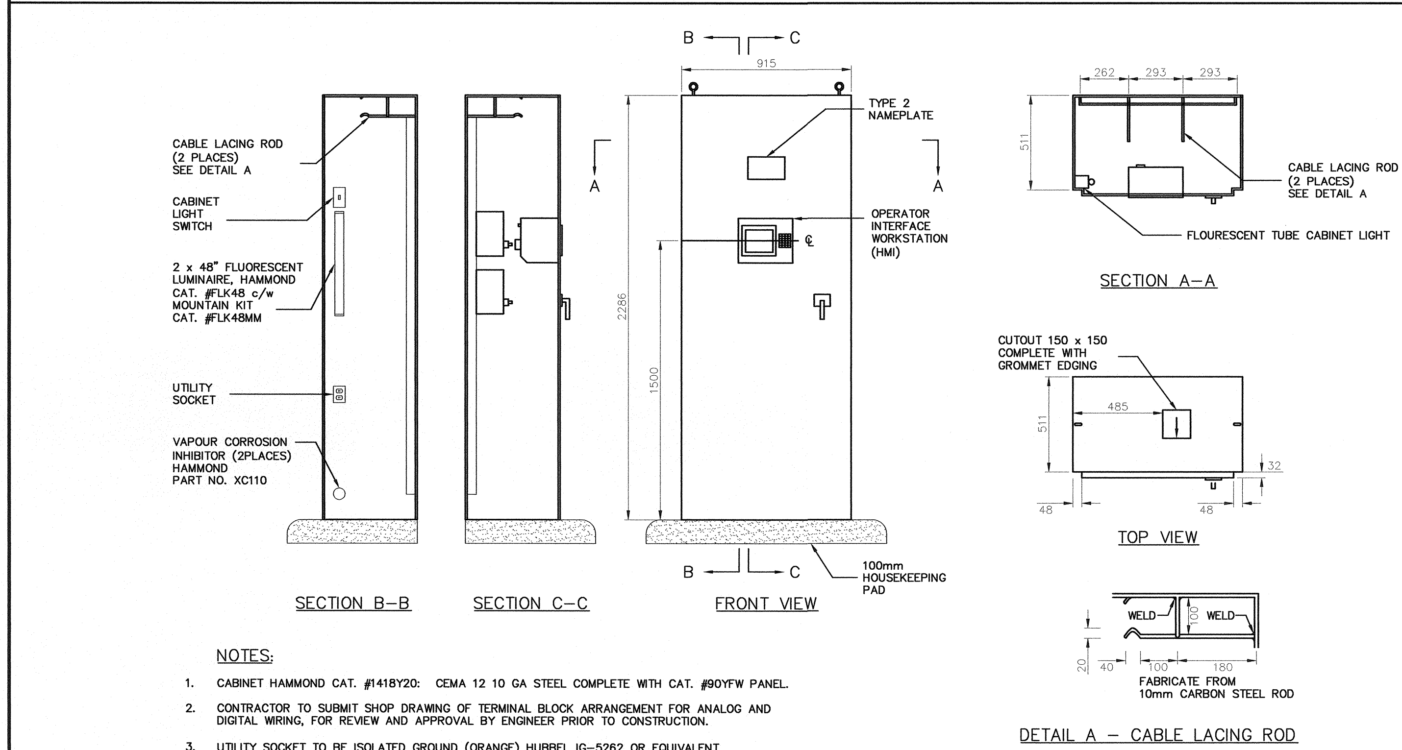
2 E5 PLC CABINET ELEVATION N.T.S.
