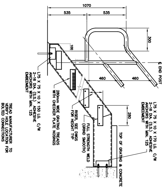
H DETAIL 1:15
