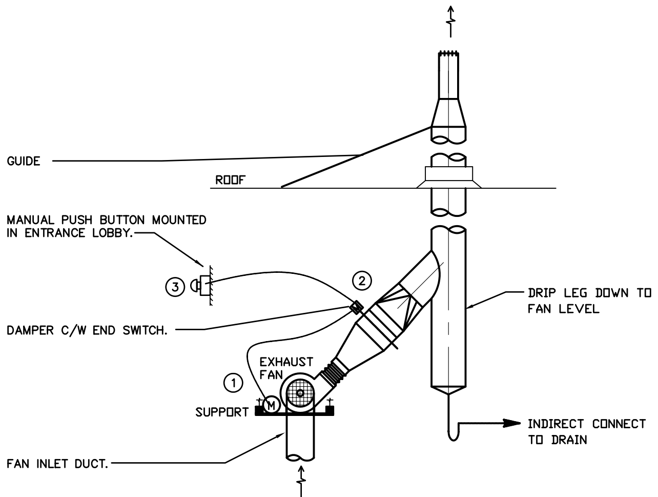
EXHAUST FAN EF-3 N.T.S.
