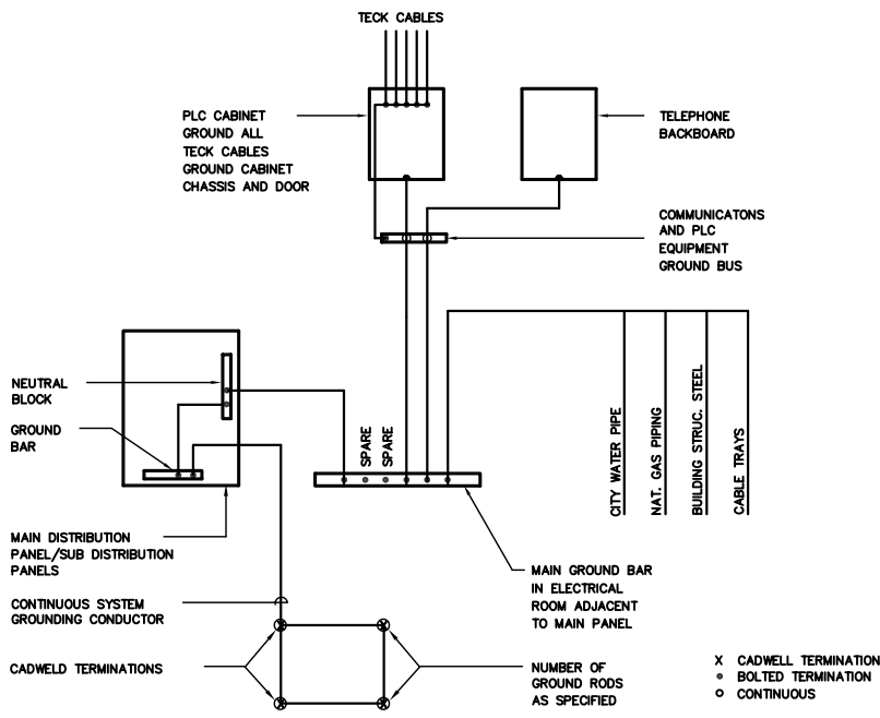
GROUNDING DETAIL N.T.S.
