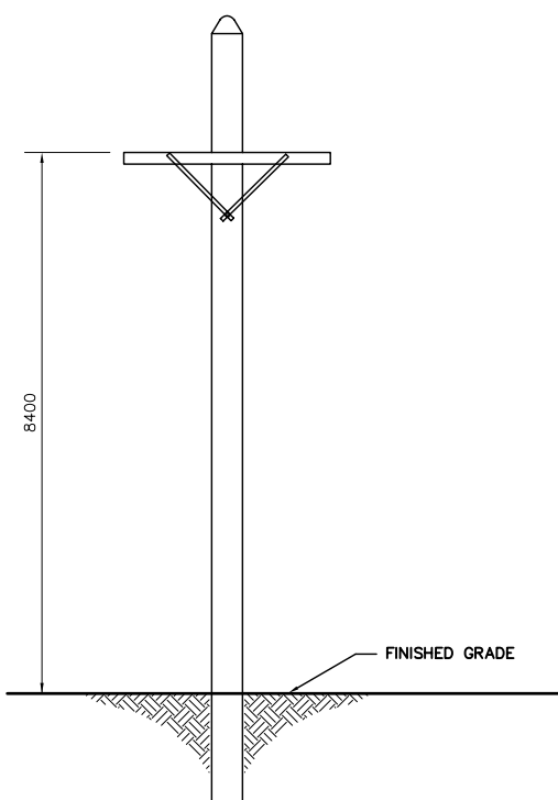
WOOD POLE DETAIL N.T.S.
