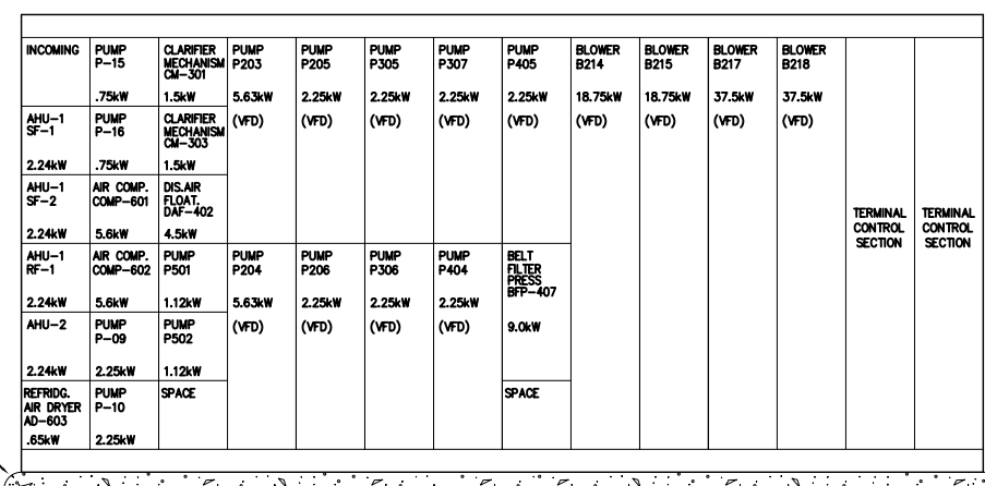
MCC-1 ELEVATION DETAIL N.T.S.
