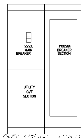
MDP ELEVATION DETAIL N.T.S.
