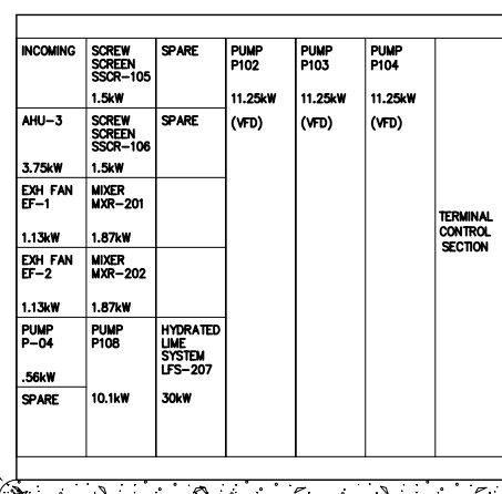
MCC-2 ELEVATION DETAIL N.T.S.
