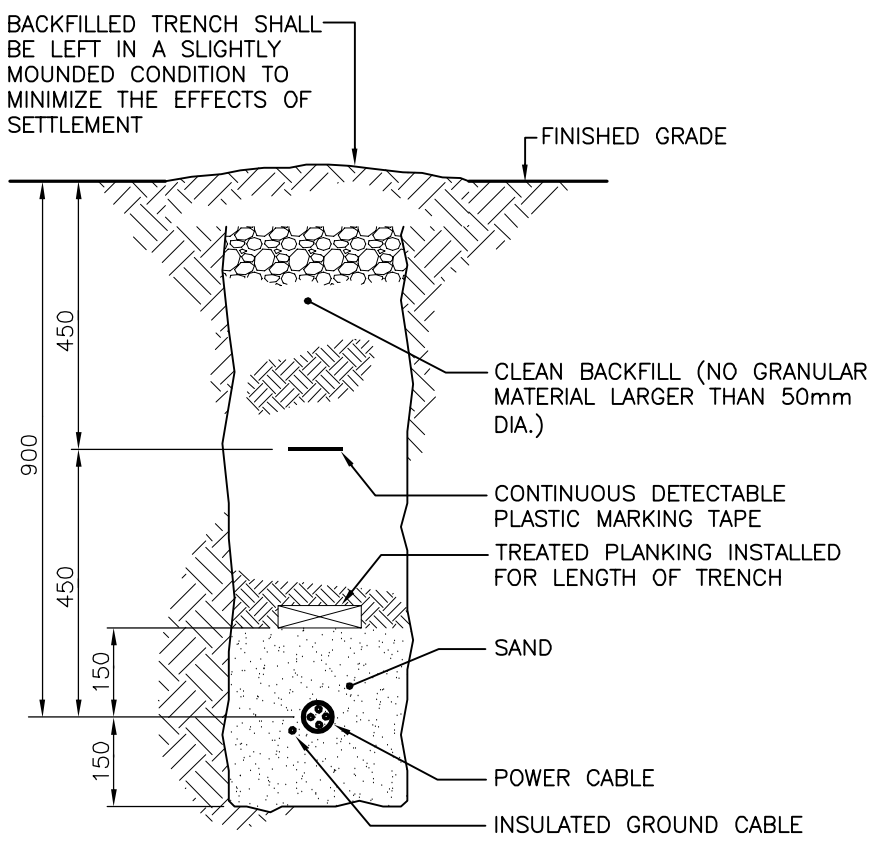
A TRENCH DETAIL N.T.S.
