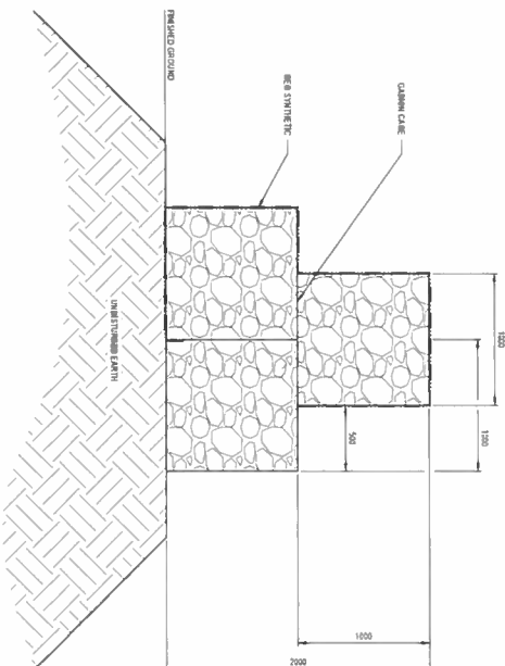
2 102 GABION 4 SCALE: 1/2"
